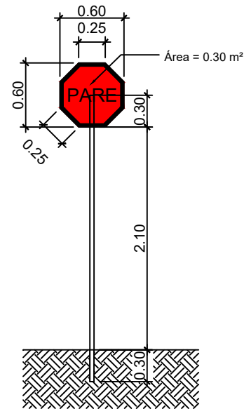
DETALHE SINALIZAÇÃO VERTICAL
