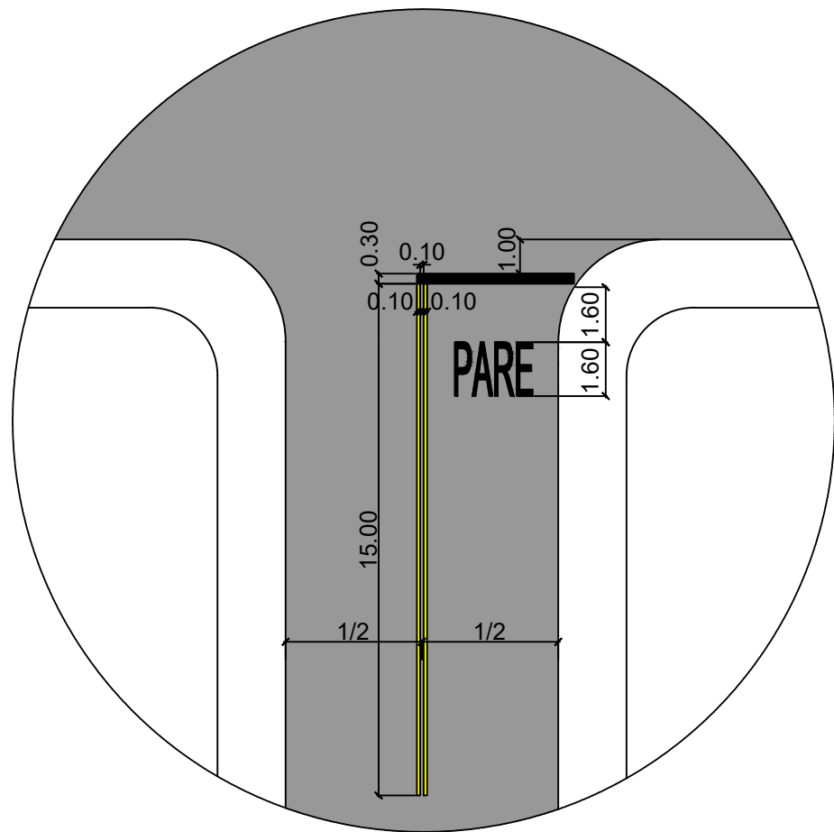
DETALHE SINALIZAÇÃO HORIZONTAL PARE
