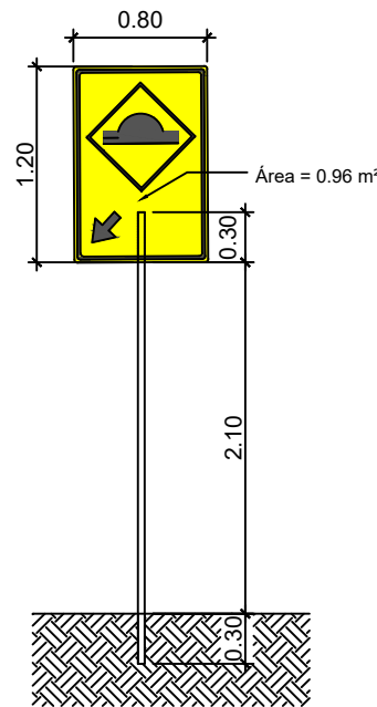
DETALHE SINALIZAÇÃO VERTICAL
