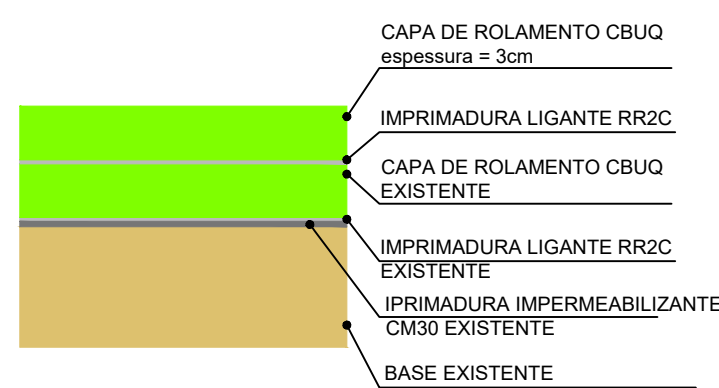
DETALHE RECAPE
